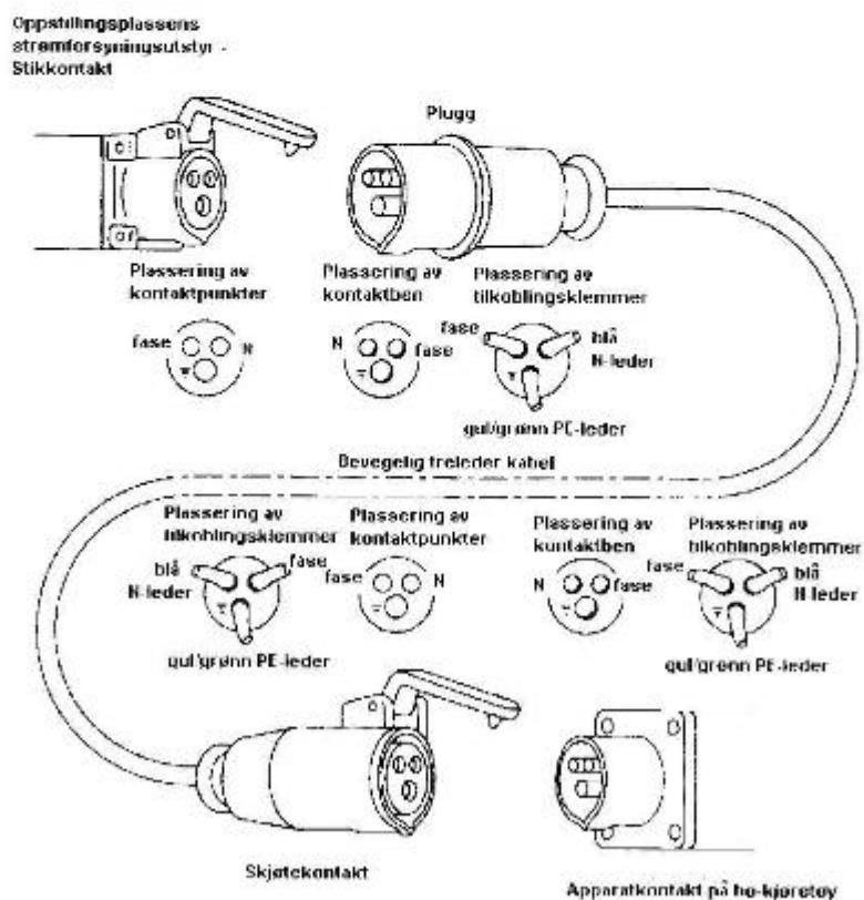
Figur 708A - Eksempel på tilkoblingskabel mellom oppstillingsplassens strømforsyningsutstyr for og fritids bo-kjøretøyet bestående av 2 poler og PE-leder.
